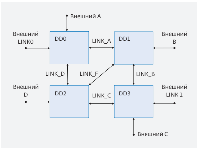
Рис.3. Схема соединения link-портов submodule
