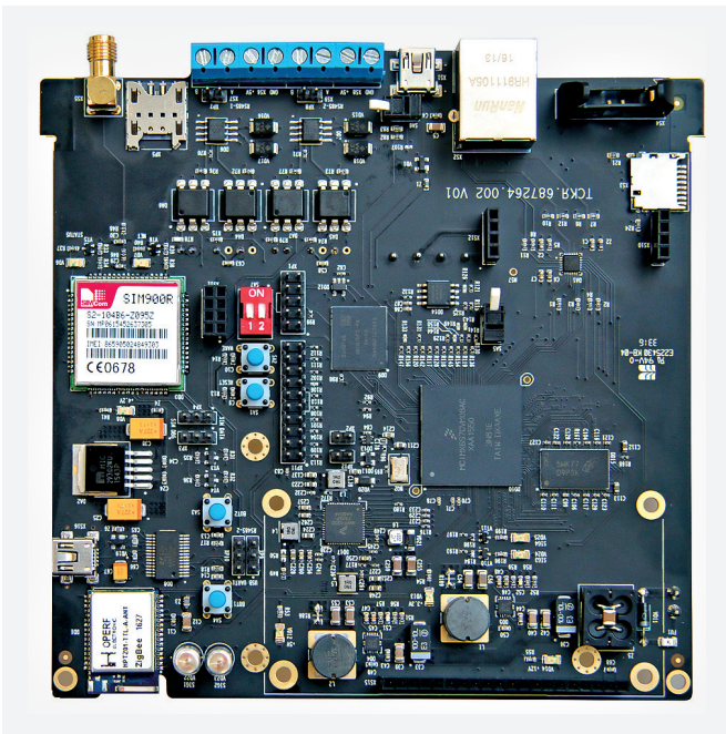
Рис.2. Собранная плата УСЦД
