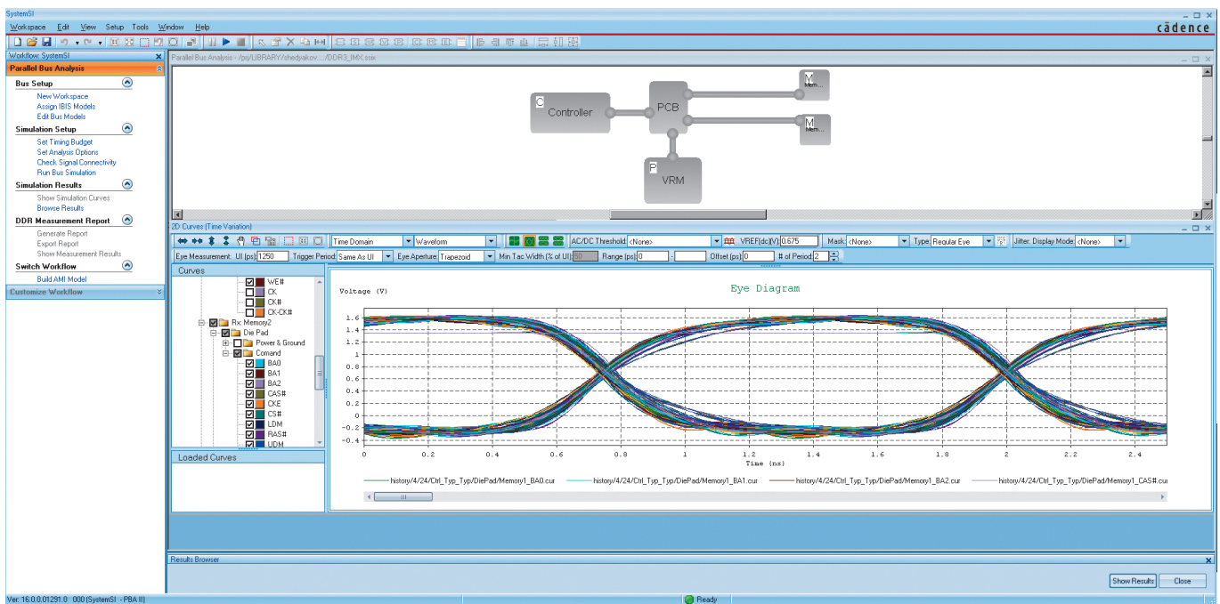
Рис.3. Глазковая диаграмма обмена данными по протоколу DDR3
