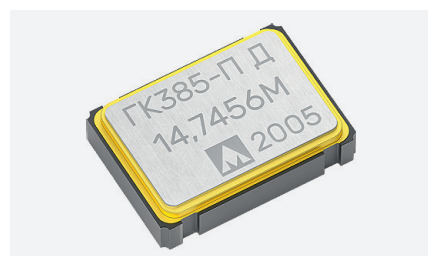
Рис. 1. Внешний вид генератора ГК385-П
